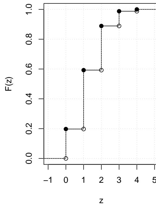
p=1/3
