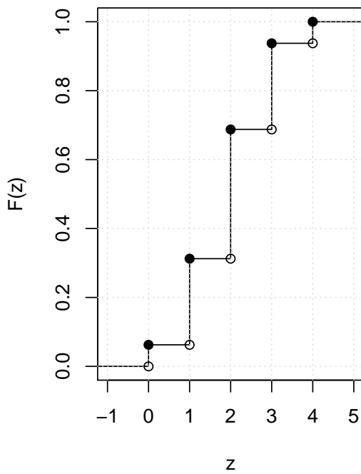
p=1/2
