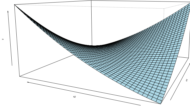
Abbildung 4.4: f(x_1, x_2) = x_1^2 - 4x_1x_2 + x_2^2 + \frac{2}{3}
