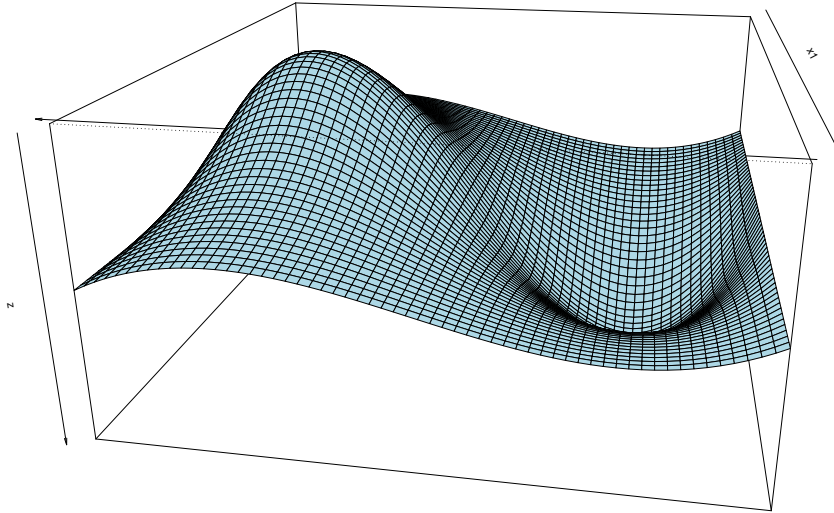
Abbildung 4.3: f(x_1, x_2) = \frac{(x_2^3 - 4x_2)}{(1 + x_1^2)}
