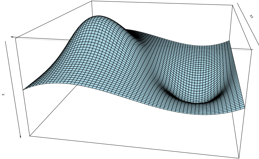
Abbildung 4.6: f(x_1, x_2) = \frac{(x_2^3 - 4x_2)}{(1 + x_1^2)}
