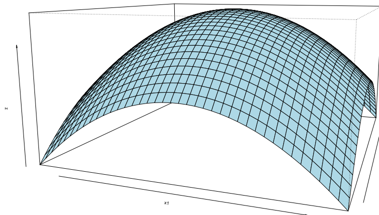
Abbildung 4.2: f(x_1, x_2) = 2 - x_1^2 - x_2^2
