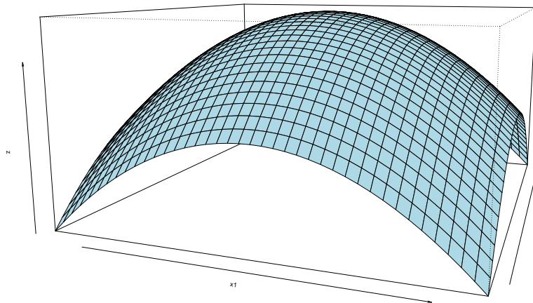
Abbildung 4.5: f(x_1, x_2) = 2 - x_1^2 - x_2^2
