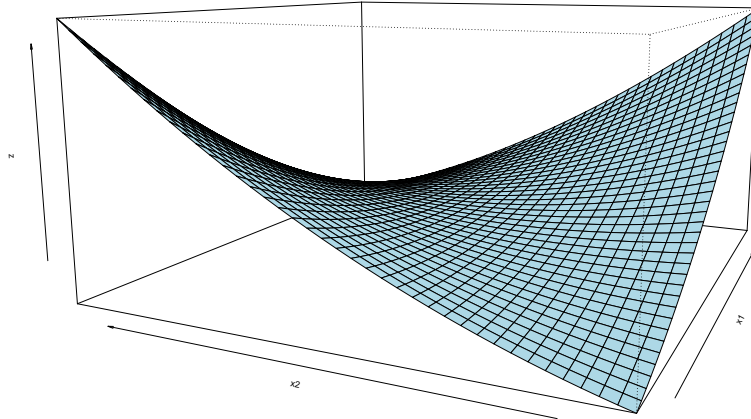
Abbildung 4.1: f(x_1, x_2) = x_1^2 - 4x_1x_2 + x_2^2 + \frac{2}{3}
